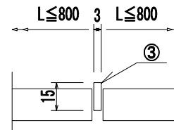
羽根分割要領 有効寸法 h
