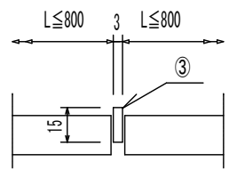
羽根分割要領 有効寸法 ω · h
