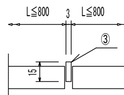
羽根分割要領 有効寸法 ω · h
