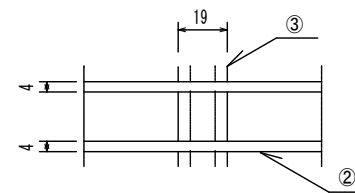
羽根補強要領 有効寸法 \omega > 800
